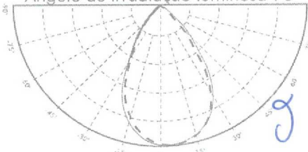
Lente de Vidro Borossilicato Ângulo de irradiação luminosa 90°
