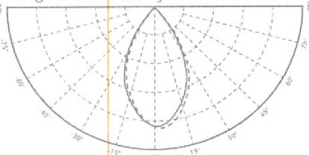
Lente de Vidro Borossilicato Ângulo de irradiação luminosa 60°
